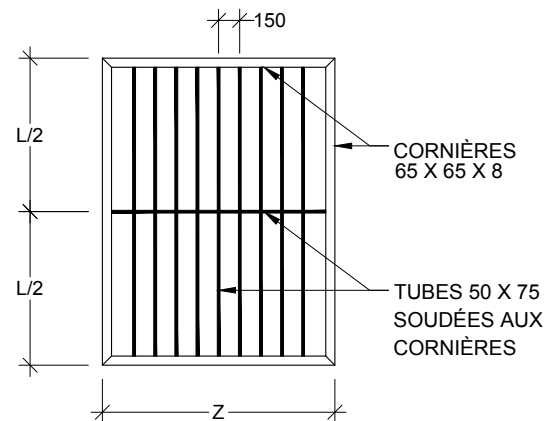
GRILLE TYPE
