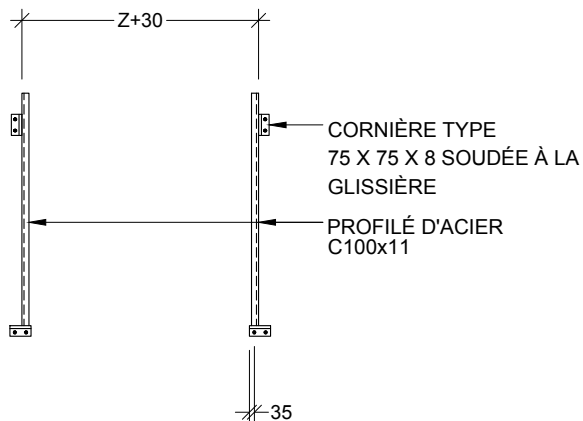
GLISSIÈRE
