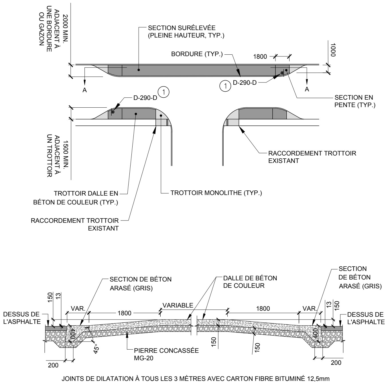
COUPE A-A AUCUNE ÉCHELLE
