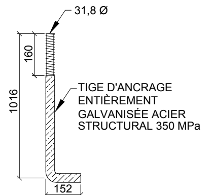
TIGE D'ANCRAGE
