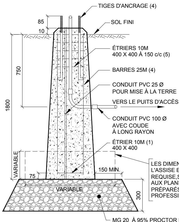
ÉLÉVATION
