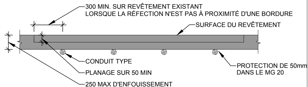
COUPE A - A'
