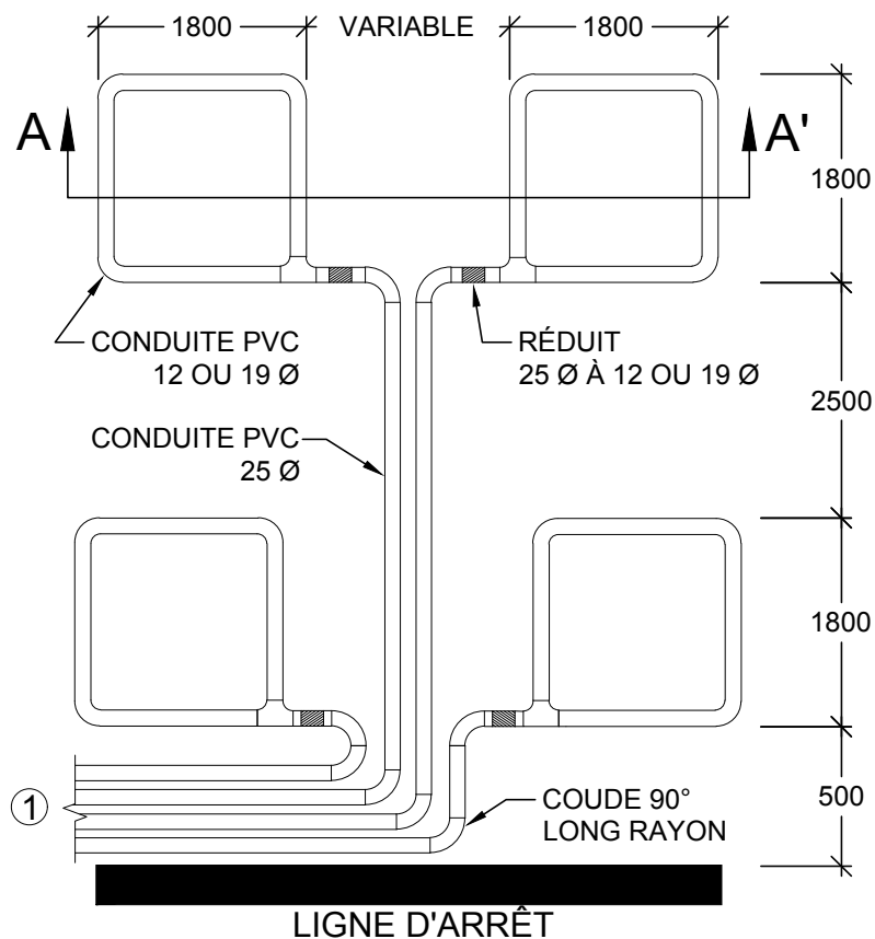
RACCORDEMENT TYPIQUE D'UNE BOUCLE DE DÉTECTION AU PUIT D'ACCÈS
