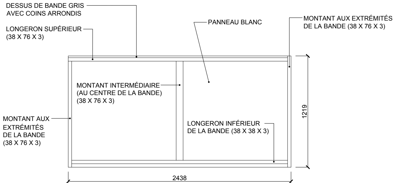
COUPE LONGITUDINALE
