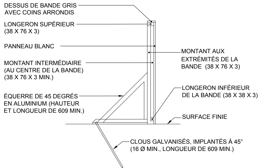
COUPE TRANSVERSALE
