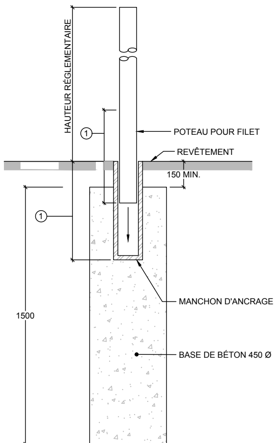
POTEAU DÉMONTABLE
