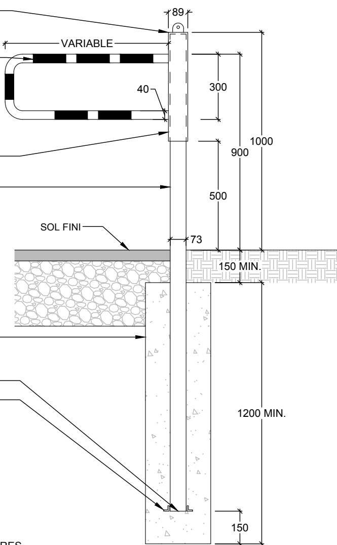
PARTIE SUPÉRIEURE DE LA SECTION PIVOTANTE
