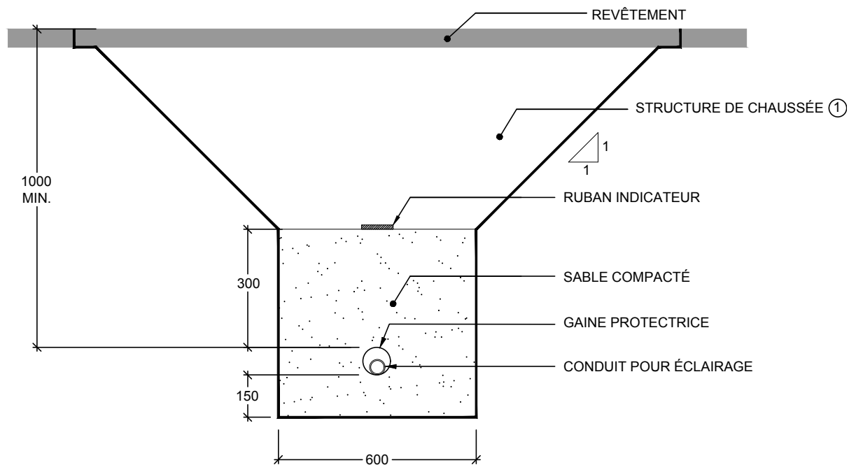
EXCAVATION DANS UNE CHAUSSEE
