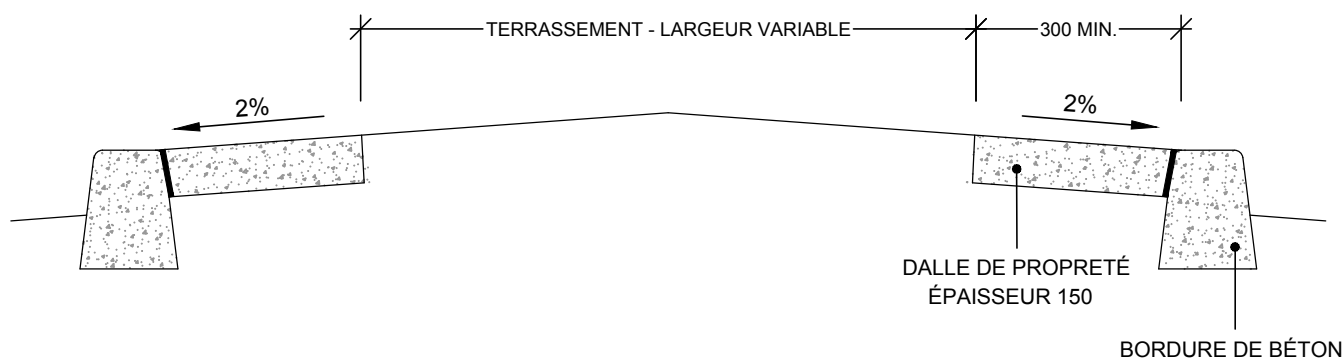
COUPE A-A'- (SITUATION 1)
