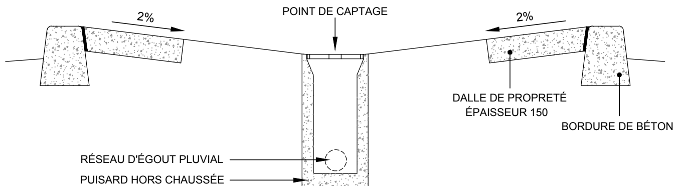
COUPE A-A'- (SITUATION 2)
