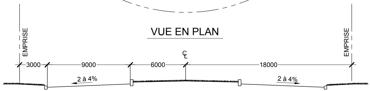
COUPE A-A'
