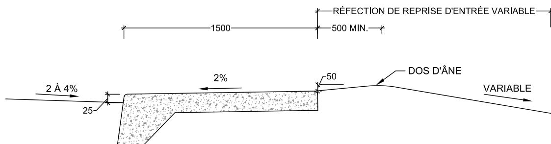
RÉFECTION AVEC TROTTOIR MONOLITHE
