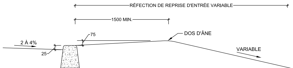
RÉFECTION AVEC BORDURE
