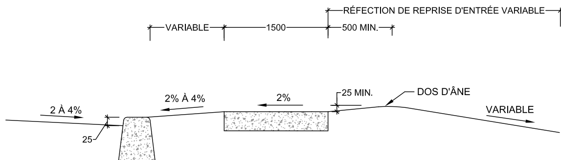
RÉFECTION AVEC BORDURE ET TROTTOIR DALLE
